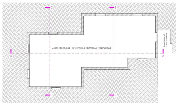
PIANO INTERRATO-INTERCAPEDINE FONDAZIONALE scala 1/100
